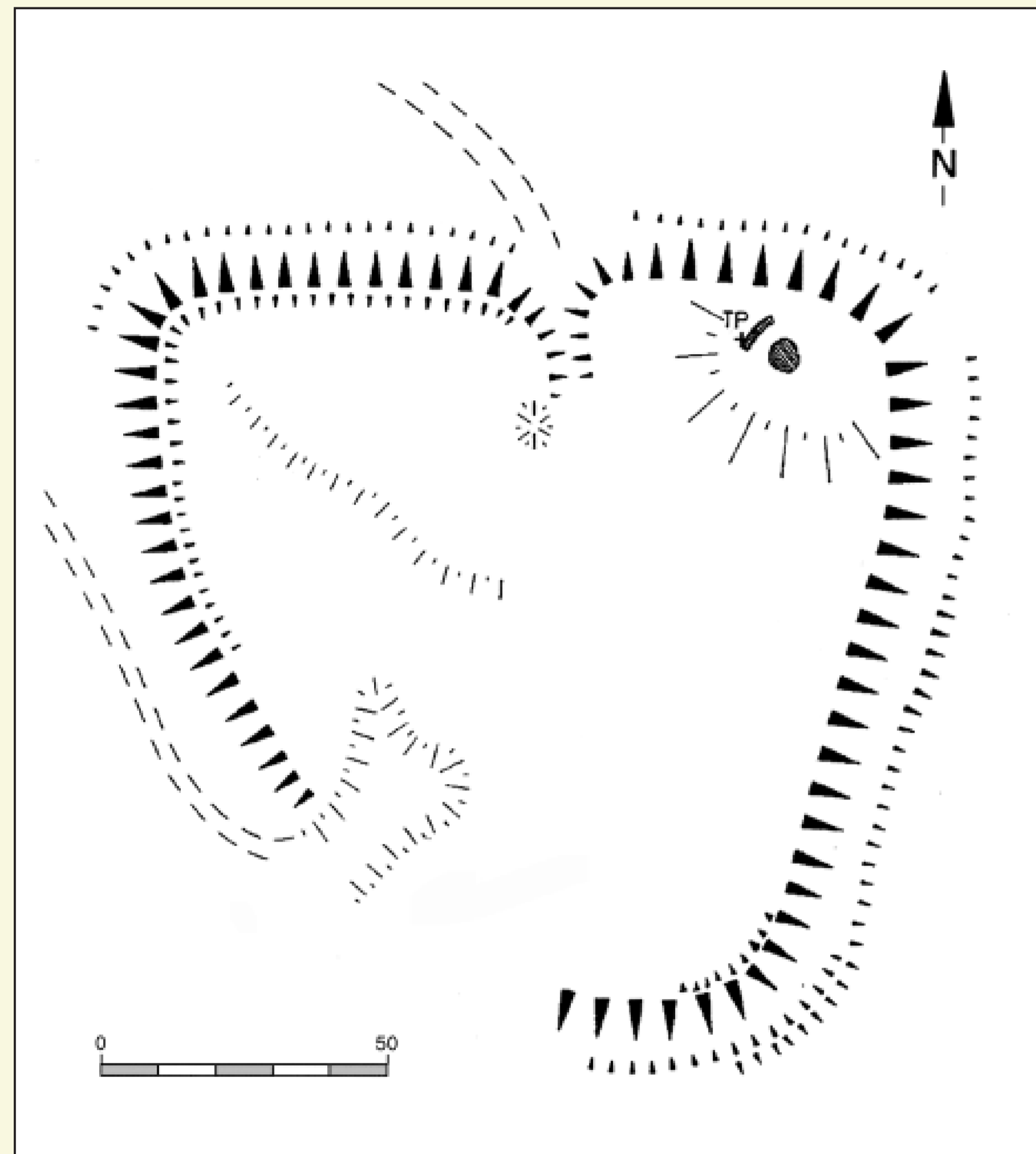
Wallanlage und Warte am Ahlberg: Der Grundriss zeigt die Wallböschung mit der Toröffnung auf der Nordseite. Auf dem Gipfelplateau sind die Fundamente der Ahlbergwarte und der Umfassungsmauer eingetragen (nach Gensen, 1986).
