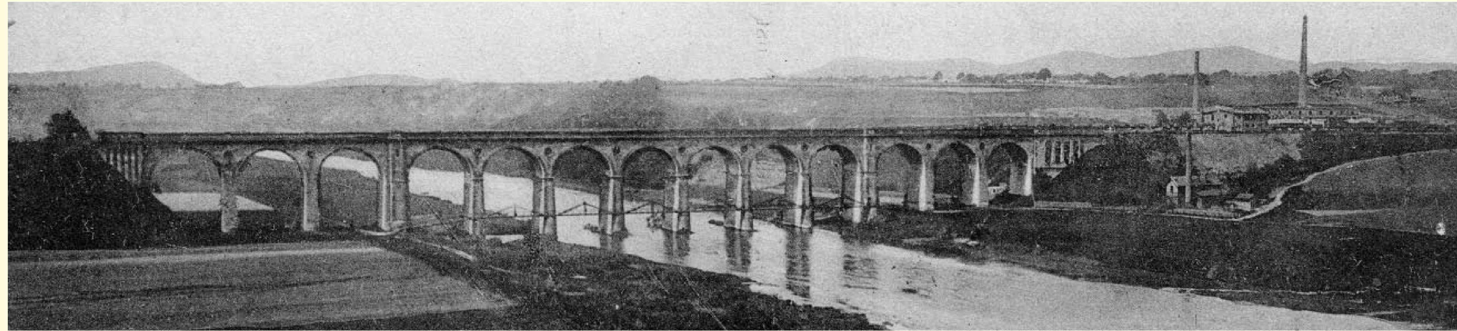
Die Gunterhäuser Eisenbahnbrücke über die Fulda um 1900. Im Hintergrund ist rechts die Ziegelei Mergard zu erkennen.
