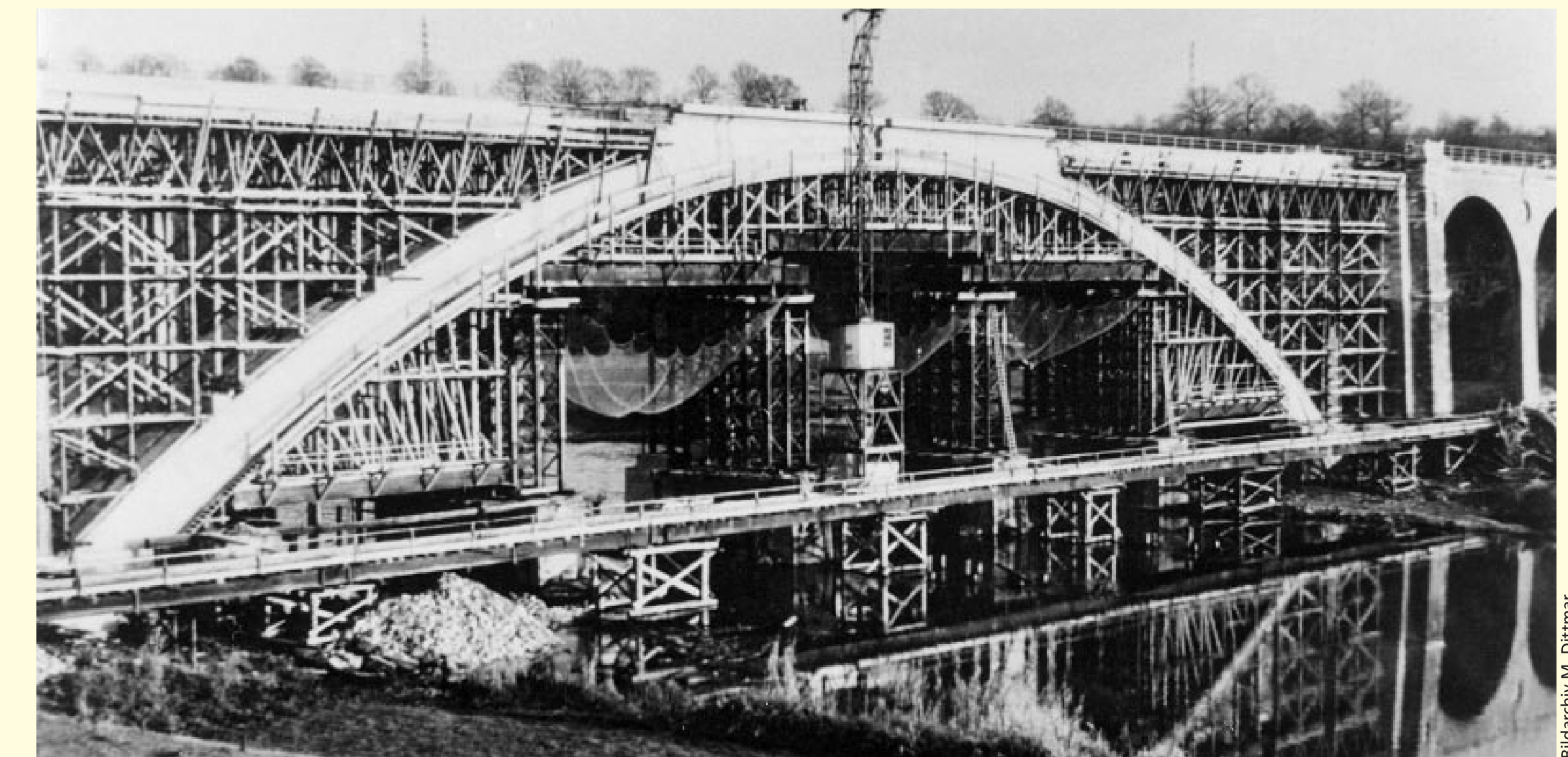
Seit 1952 überspannt ein einzelner Bogen die Fulda.
